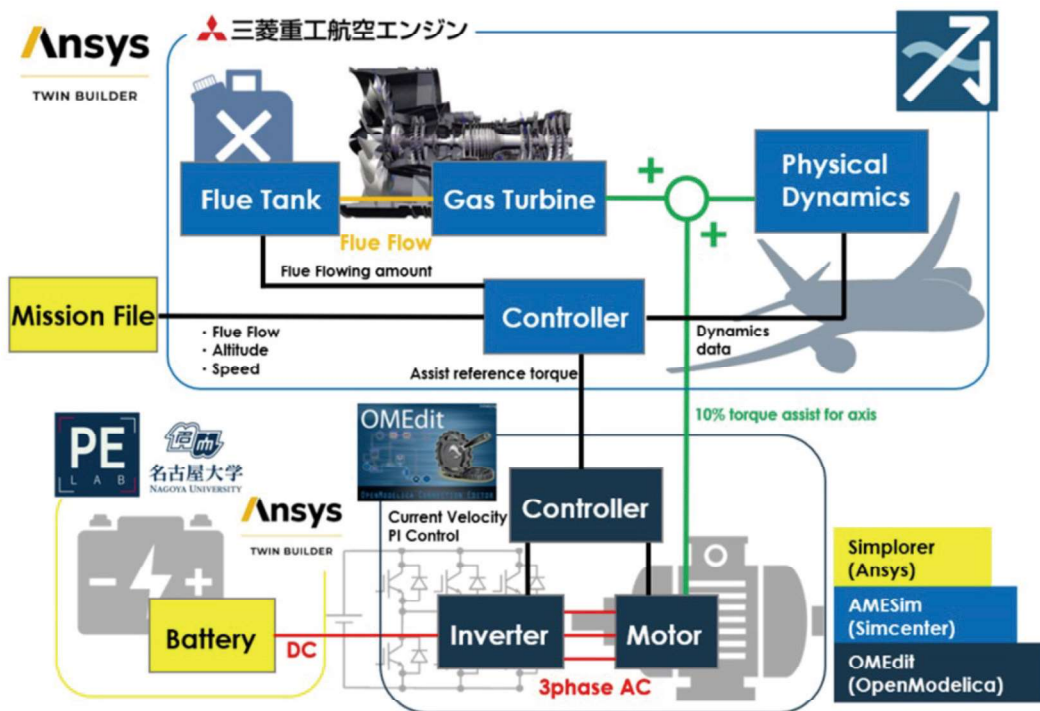
電気系統と機械／油圧系統の連成解析
