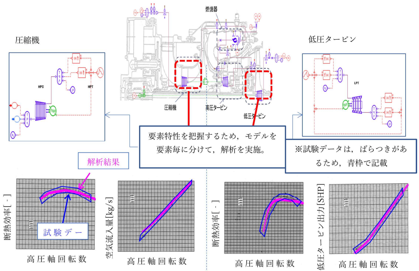
ガスタービンエンジンのシミュレーション概要
